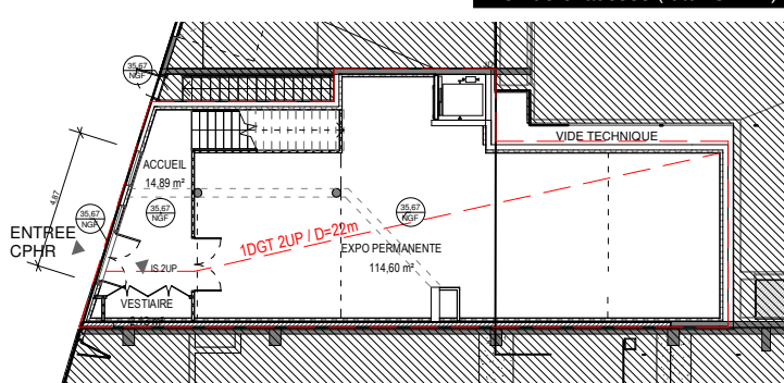
Rez-de-chaussée (futur CPHR)
