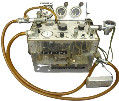
Respirateur RPN (Rosenstiel-Pesty-Rosenthal) conçu en 1955, à l'instigation de Maurice Cara, professeur d'anesthésie à l'hôpital Necker-Enfants Malades à Paris. Coll. CPHR
